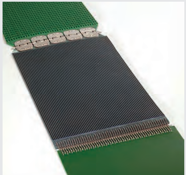
Mechanische Verbinder
